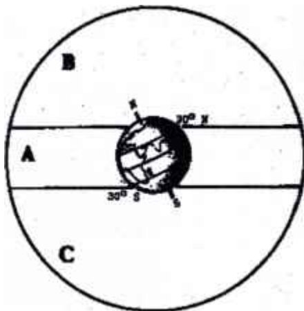
Fig 95. Sfera Celestă
